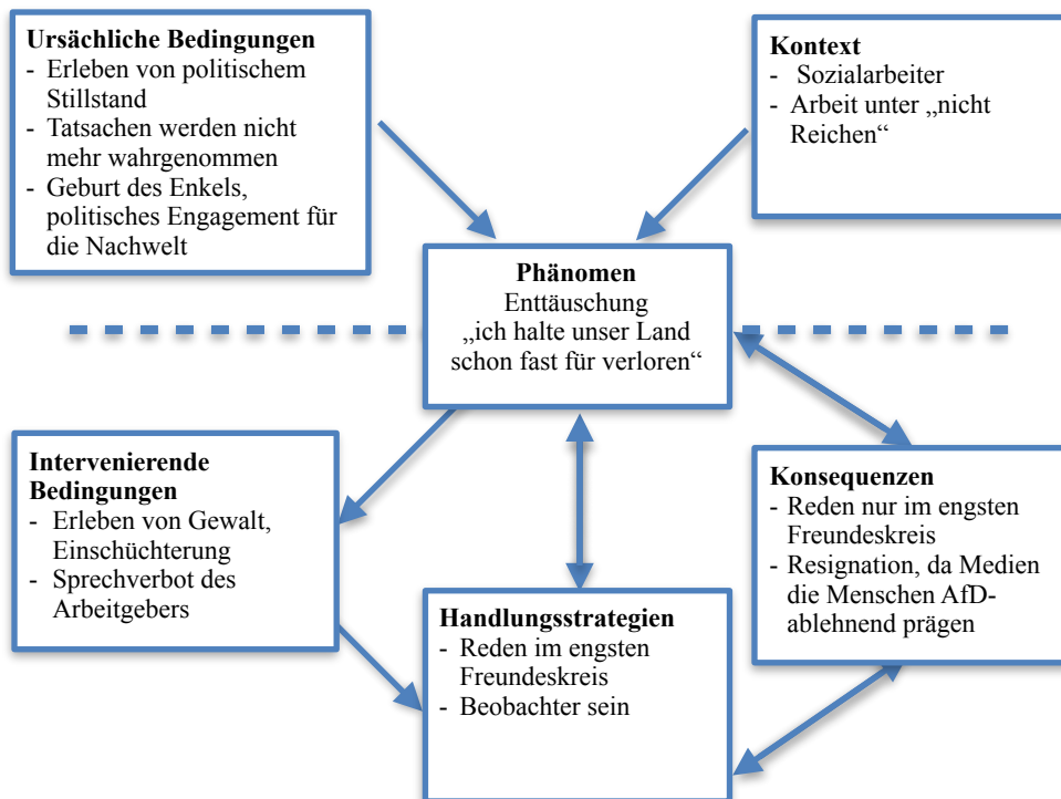
Abbildung 5: Kodierparadigma Roland
