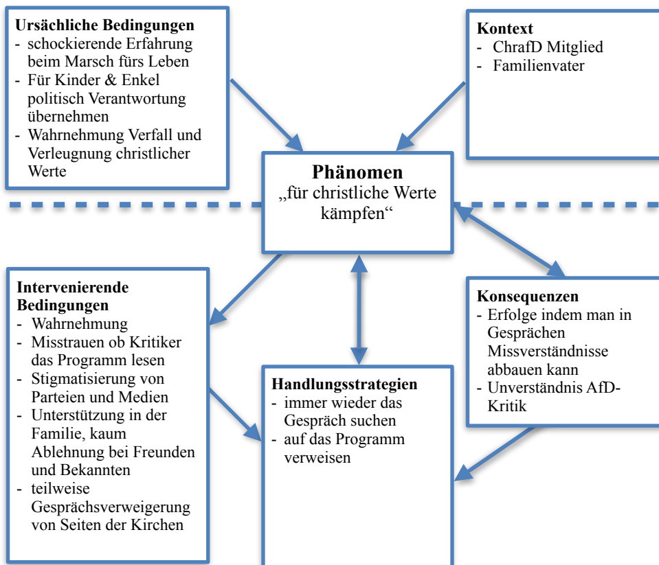
Abbildung 11: Kodierparadigma Jörg
