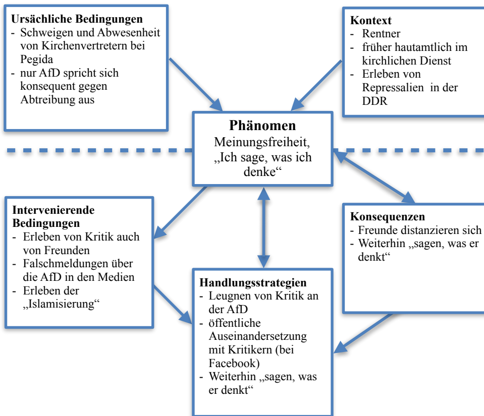
Abbildung 10: Kodierparadigma Hans
