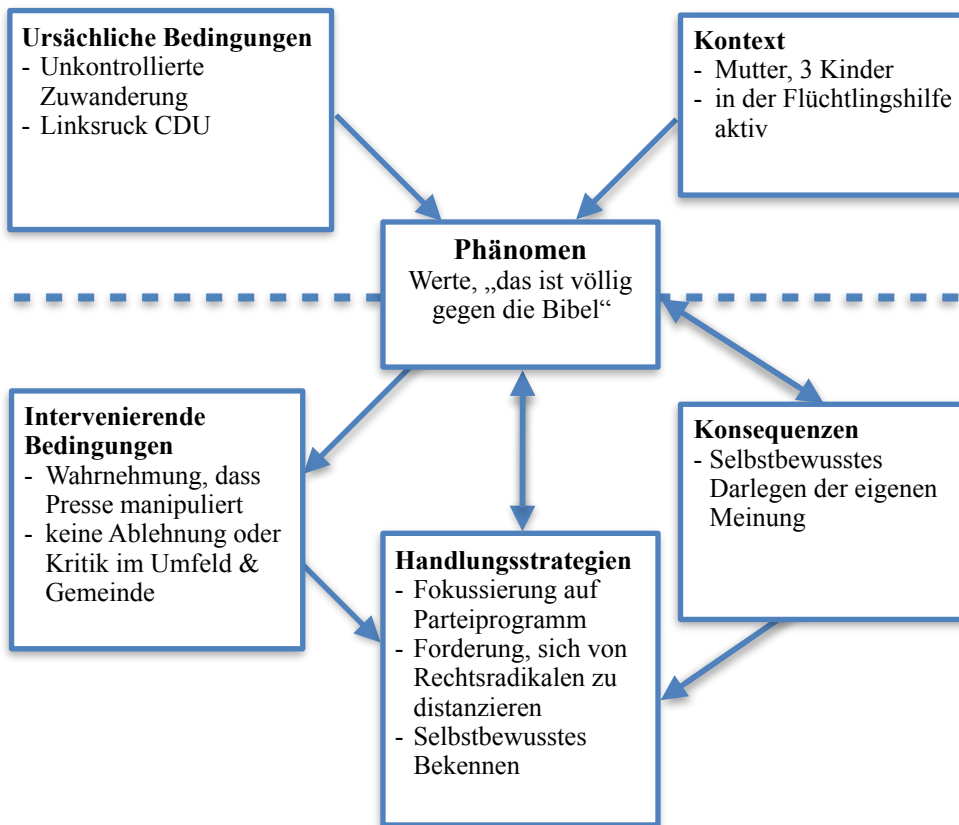
Abbildung 8: Kodierparadigma Tina
