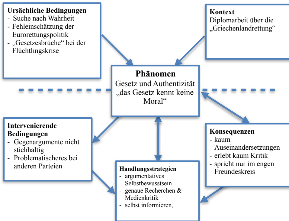
Abbildung 4: Kodierparadigma Sören
