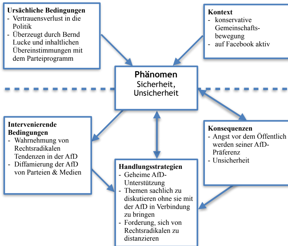
Abbildung 9: Kodierparadigma Günther
