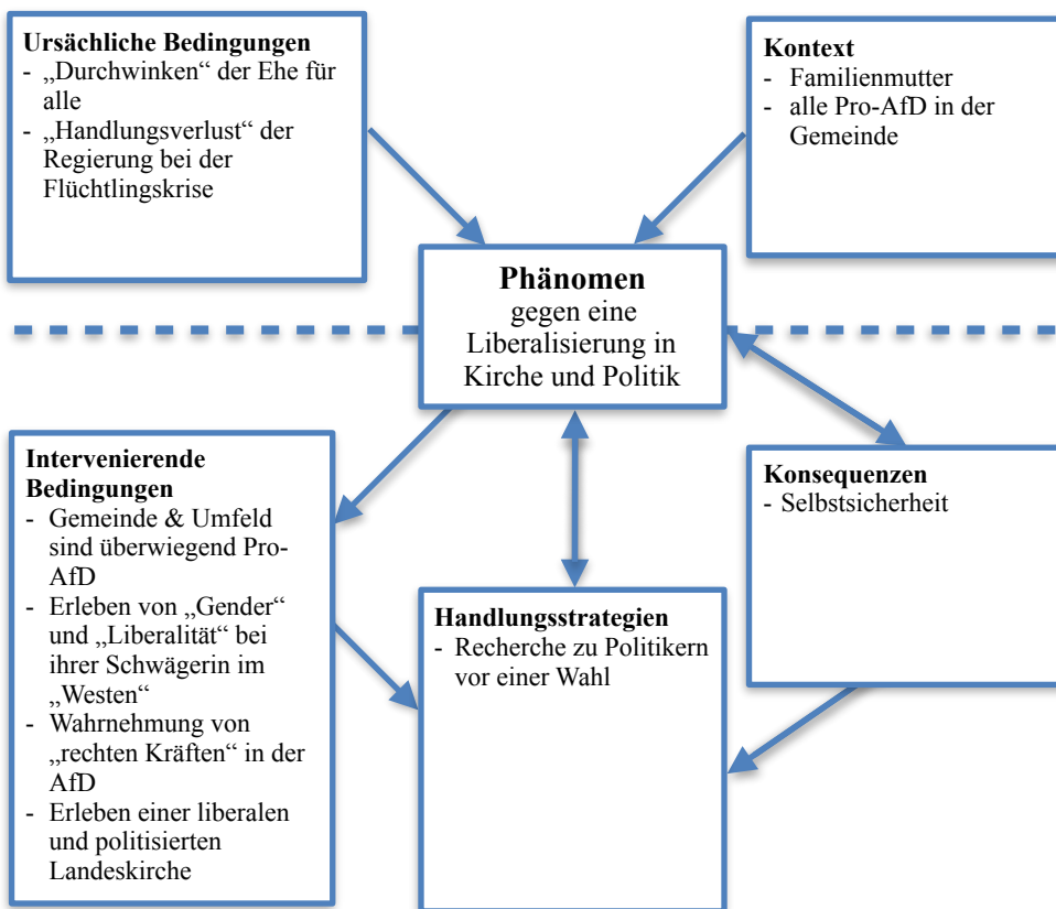
Abbildung 13: Kodierparadigma Sabrina
