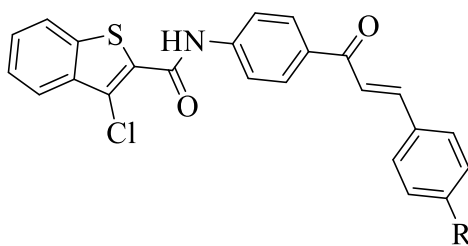
21: R = H (a), OCH 3 (b)
